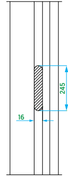
Kanat Montaj Kesiti
