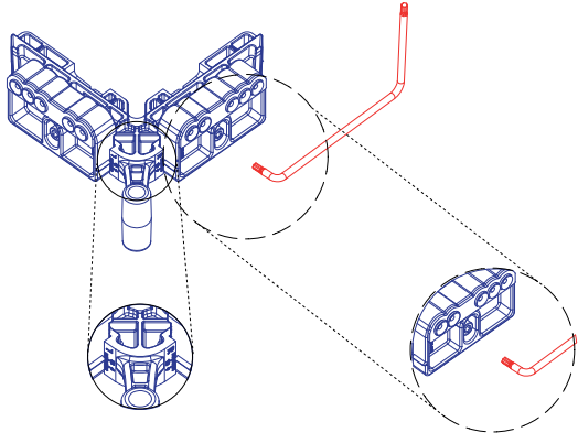
Kanat Alt Menteşe Şablonu 12/20-22 Ø3 ya da 12/18-20-22 Ø6
