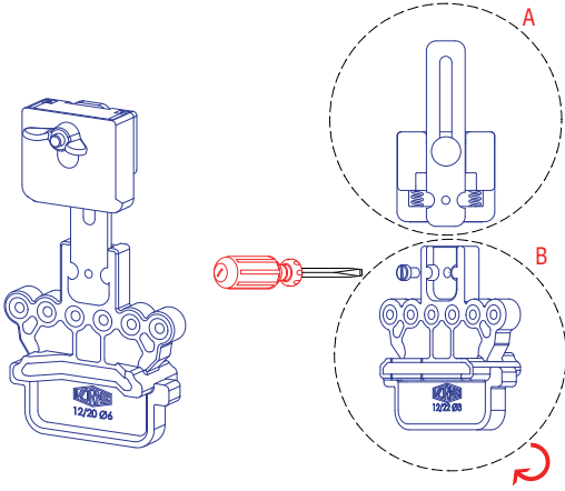
Kasa Menteşe Şablonu 12/20-22 Ø3 ya da 12/18-20-22 Ø6
